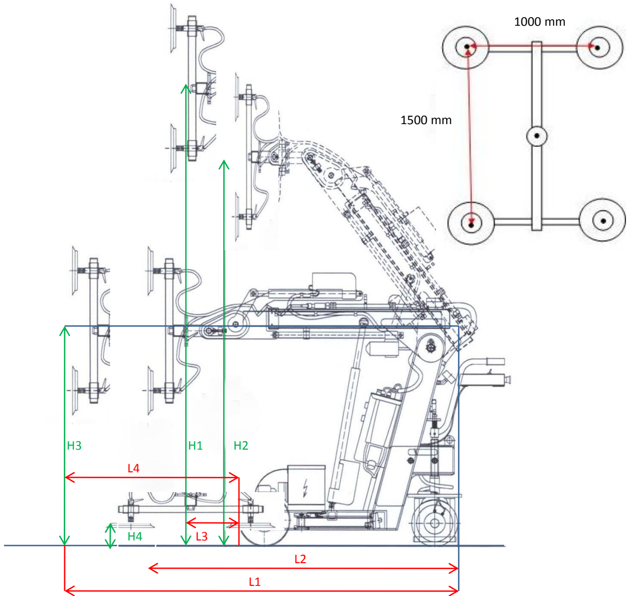
Målskema MAXI 500kg med \varnothing 360 sugekopper.
